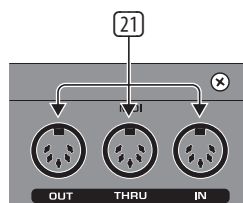
Рис. 3.5: Разъемы FBQ2496 для подключения MIDI
