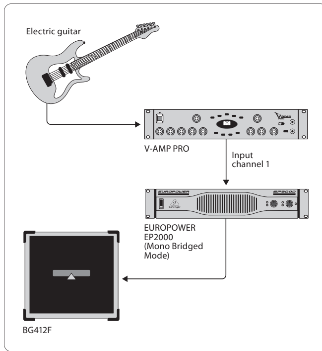
Рис. 3.5: Мостовой режим
